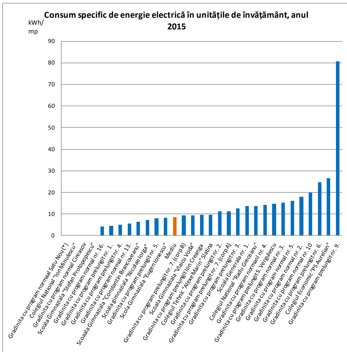
Figura 53. Consumul specific de energie electrică în unitățile de învățământ, anul 2015.
