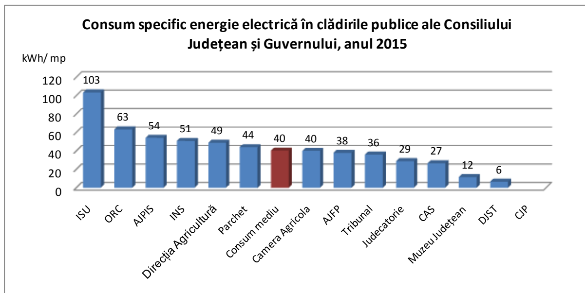
Figura 63. Consum specific energie electrică în clădirile publice ale Consiliului Județean și Guvernului, anul 2015.
