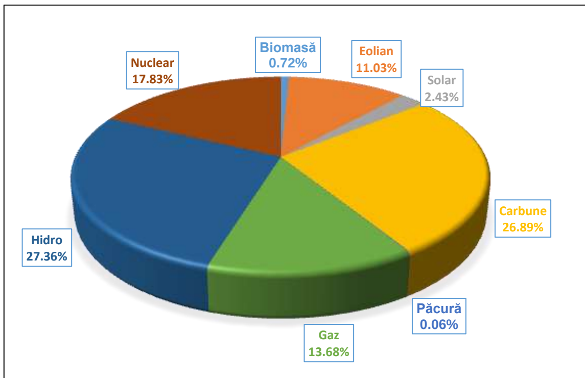
Figura 10. Structura pe tipuri de resurse a energiei electrice livrate în rețele de producători dispecerizabili și nedispecerizabili în anul 2015.
