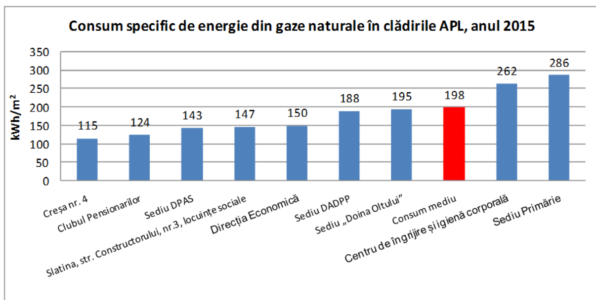
Figura 56. Consumul specific energie din gaze naturale în clădirile APL, anul 2015.
