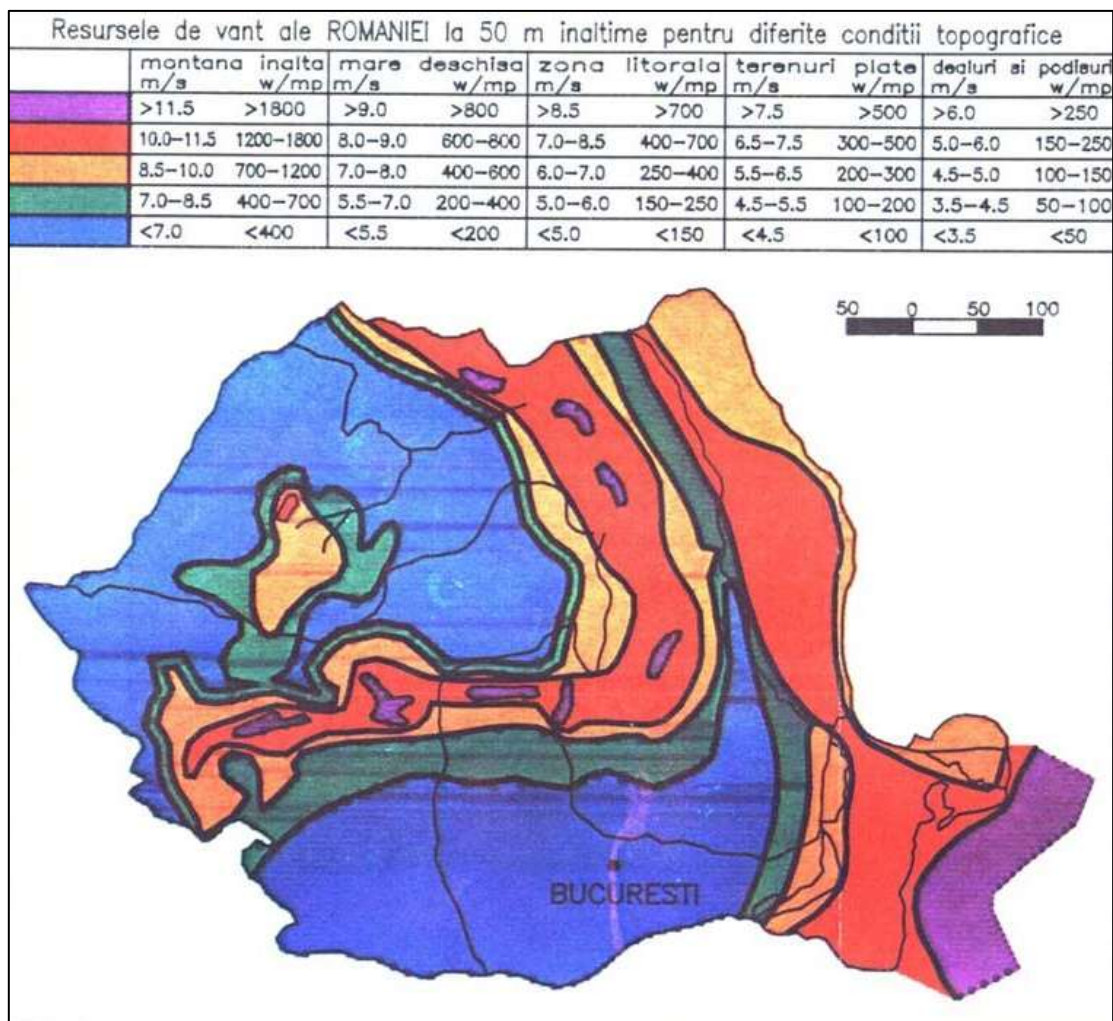
Figura 15. Resursele de vânt ale României la 50 m înălțime pentru diferite condiții topografice.
