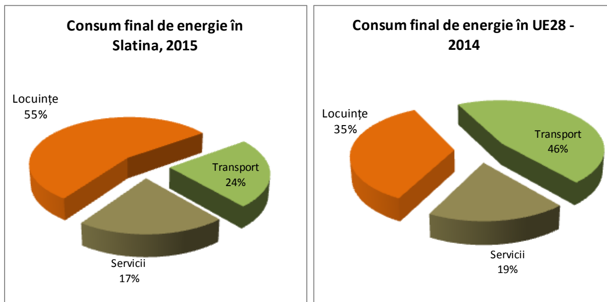
Figura 40. Comparație consum final de energie Slatina (2015) – UE28 (2014) .
