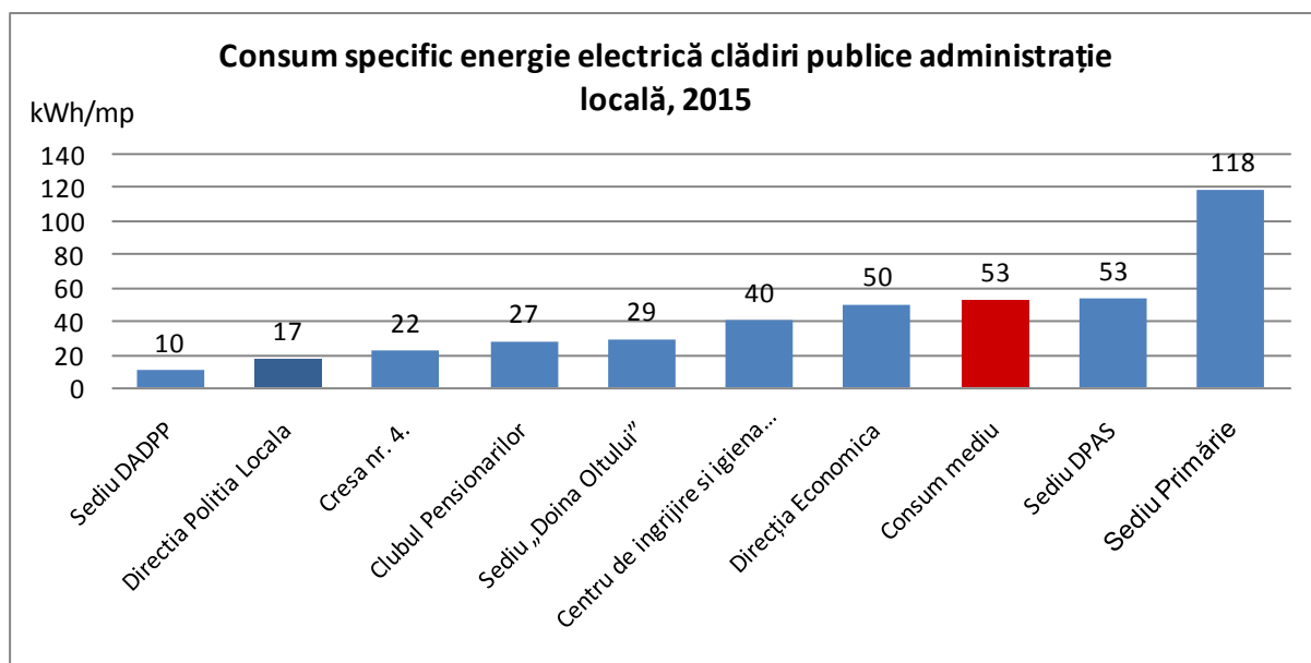
Figura 55. Consumul specific de energie electrică clădiri publice administrație, anul 2015.
