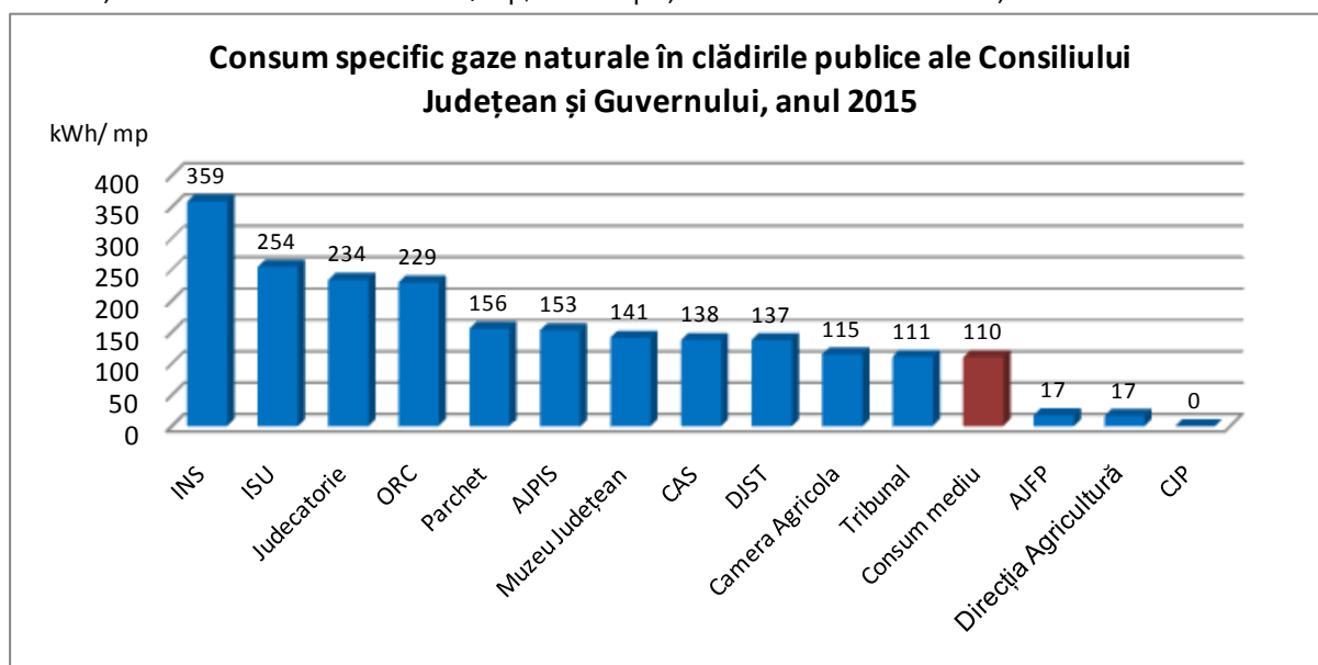
Figura 64. Consum specific gaze naturale în clădirile publice ale Consiliului Județean și Guvernului, anul 2015.
