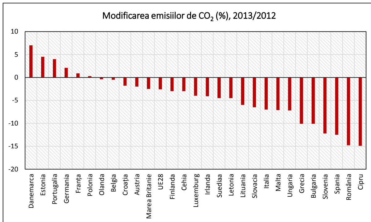
Figura 9. Modificarea emisiilor de CO 2 , 2013/2012.
