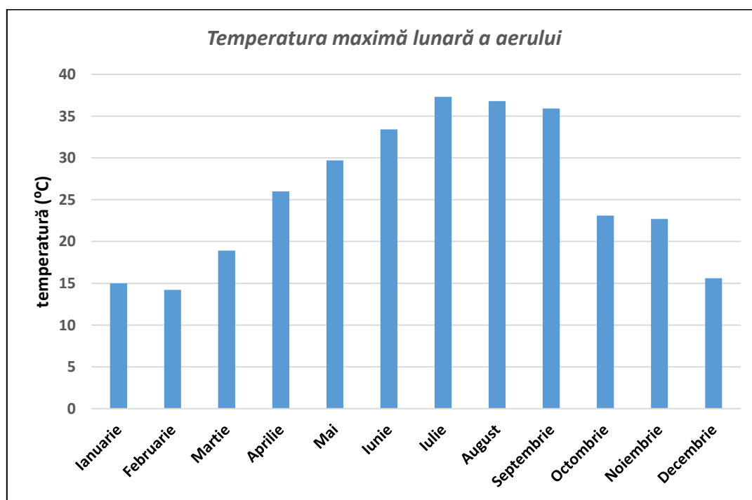
Figura 16. Evoluția temperaturilor maxime lunare înregistrate la stația meteorologică Slatina.
