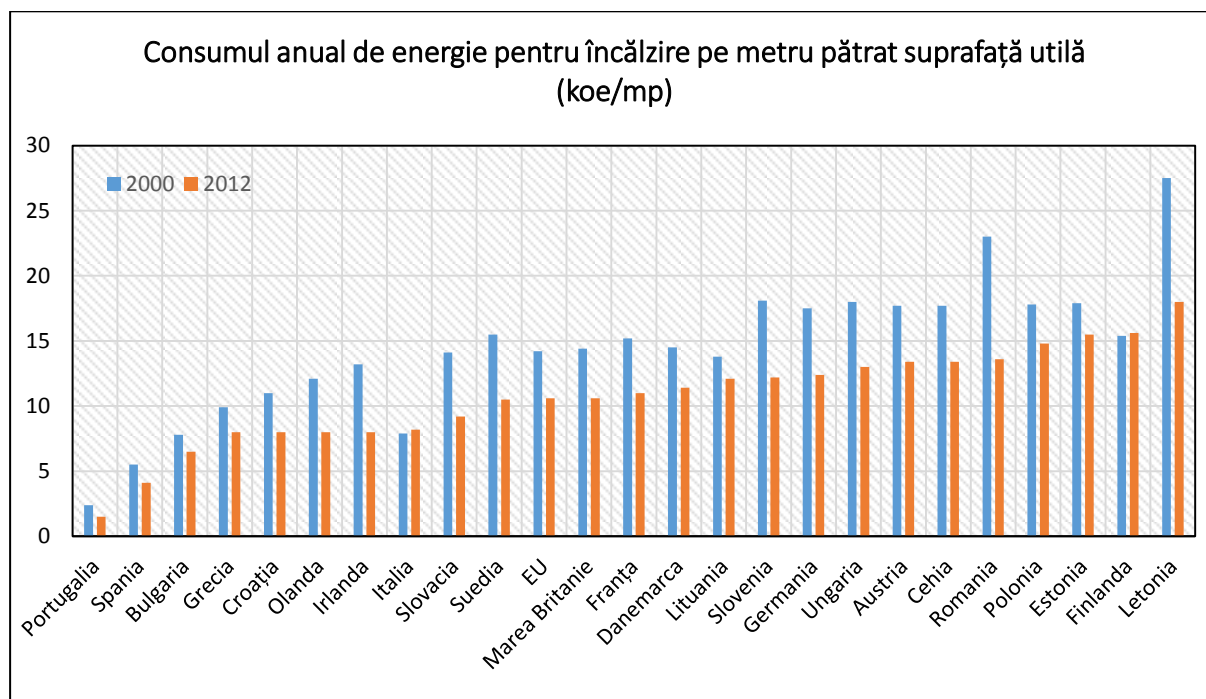
Figura 8. Consumul anual de energie pentru încălzire pe metru pătrat suprafață utilă.
