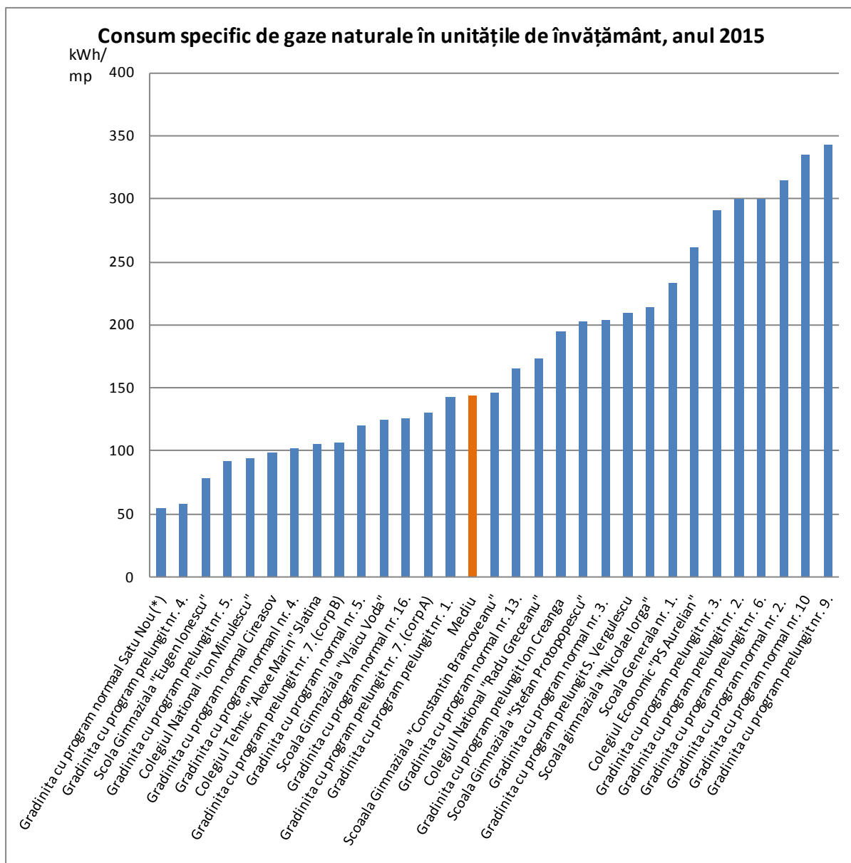
Figura 54. Consumul specific de gaze naturale în unitățile de învățământ, anul 2015.
